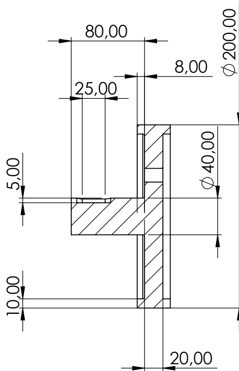
SEZIONE A-A SCALA 1 : 4
